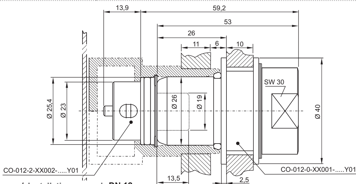
Пример установки / Installation example DN 12
