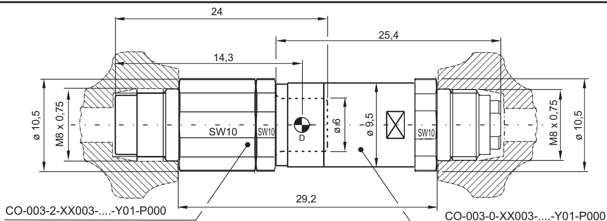
Пример установки / Installation example DN 3
